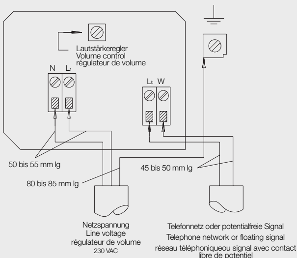
Abb. 1 / Fig. 1 Anschlussplan / Wiring diagram / Schéma de raccordement
